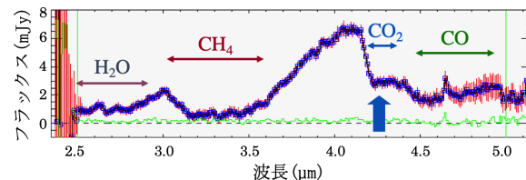
図1 画像に変換した図の例（褐色矮星のスペクトル）
